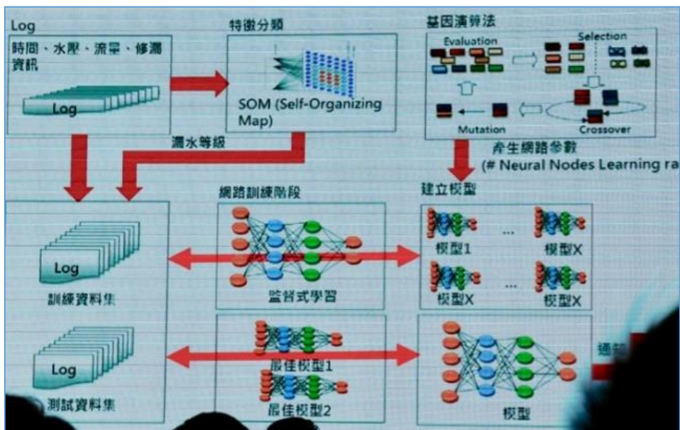
漏水預測演算法架構圖
